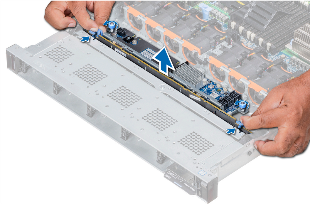
그림 59. 하드 드라이브 후면판 분리
