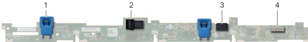
그림 60. 4 X 3.5 하드 드라이브 후면판
