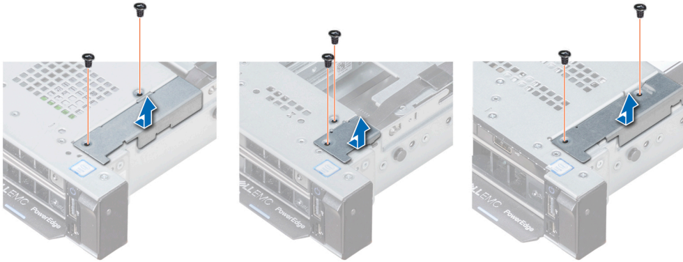
그림 79. 케이블 덮개 분리
