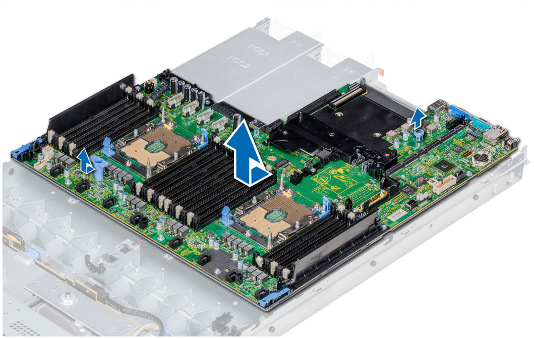
그림 72. 시스템 보드 제거
