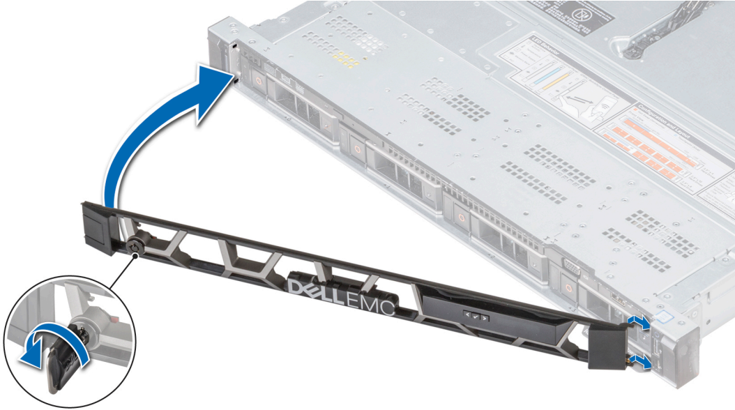
그림 15. LCD 패널이 포함된 전면 베젤(선택 사항) 설치
