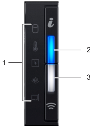
그림 3. iDRAC Quick Sync 2.0 표시등(선택 사항)이 포함된 왼쪽 제어판
