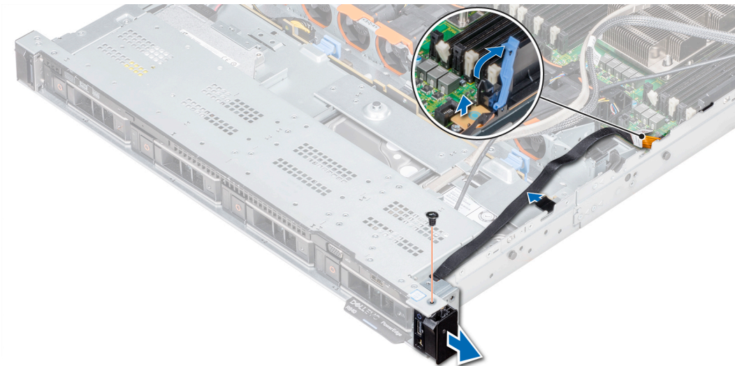
그림 80. 오른쪽 제어판 분리
