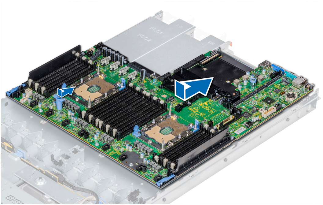
그림 73. 시스템 보드 설치
