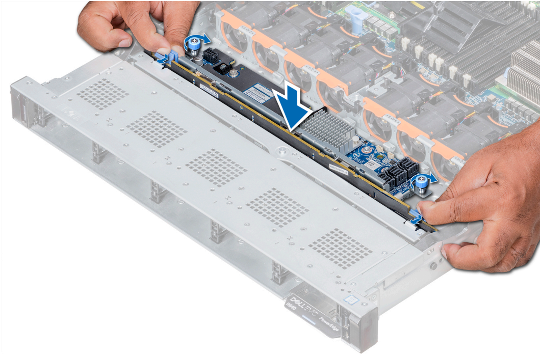
그림 61. 하드 드라이브 후면판 설치
